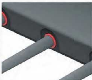
Vastag falú villa-hordozó cső, hegesztett kúpos hüvelyekkel
